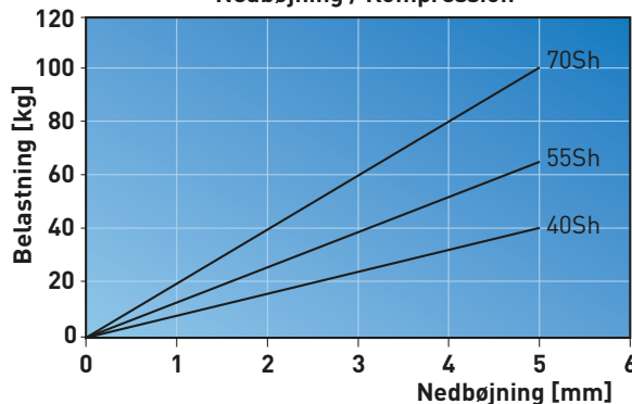
Nedbøjning / Kompression
